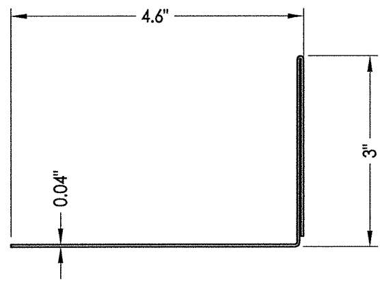
37 SILL PAN
