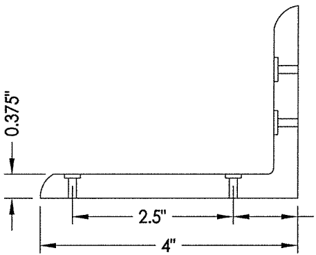
32 L-BRACKET
