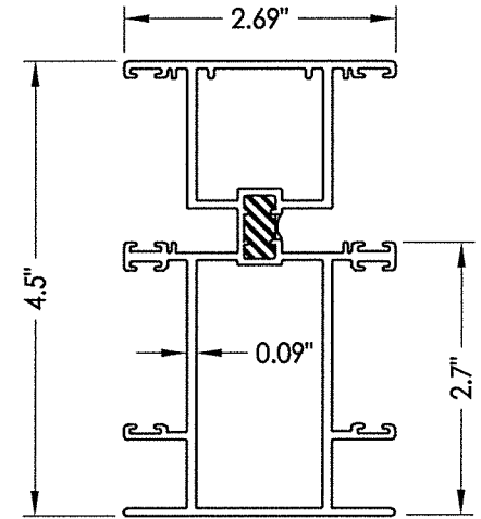
12 FALL JAMB
