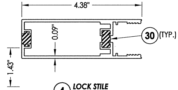
4 LOCK STILE
