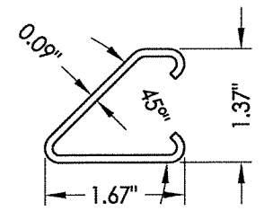
18 135° YOKE
