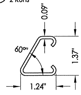
17 60° YOKE
