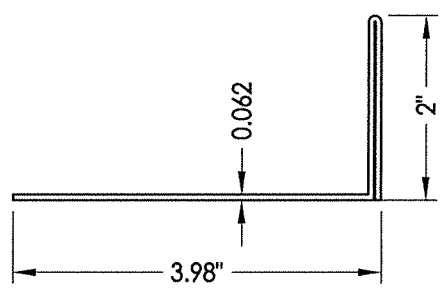
4 SILL PAN
