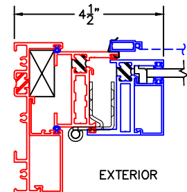
⑦ BLOCK JAMB
