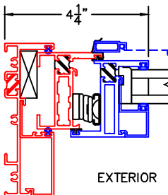
⑧ BLOCK JAMB
