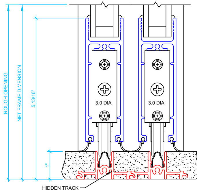
2 DOOR SILL SCALE: 6" = 1'
