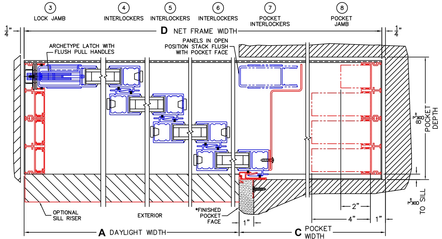
XXXXP DOOR SHOWN
