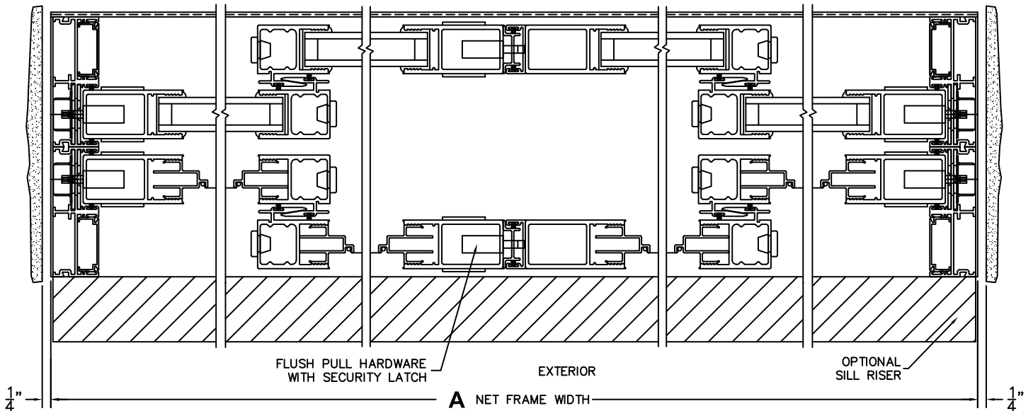
3 LOCK JAMB
