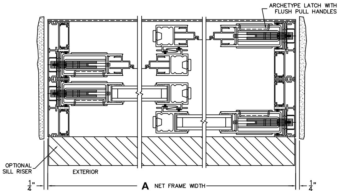
3 LOCK JAMB
