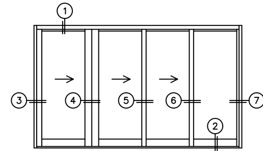
XIXXO DOOR SHOWN
