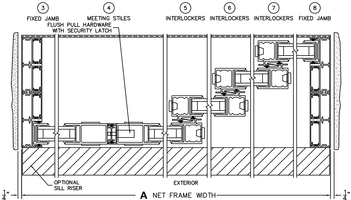
OIXXXX DOOR SHOWN
