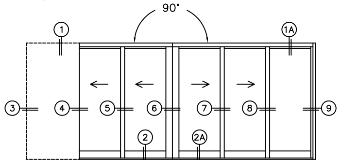
PXXIXXO DOOR SHOWN
