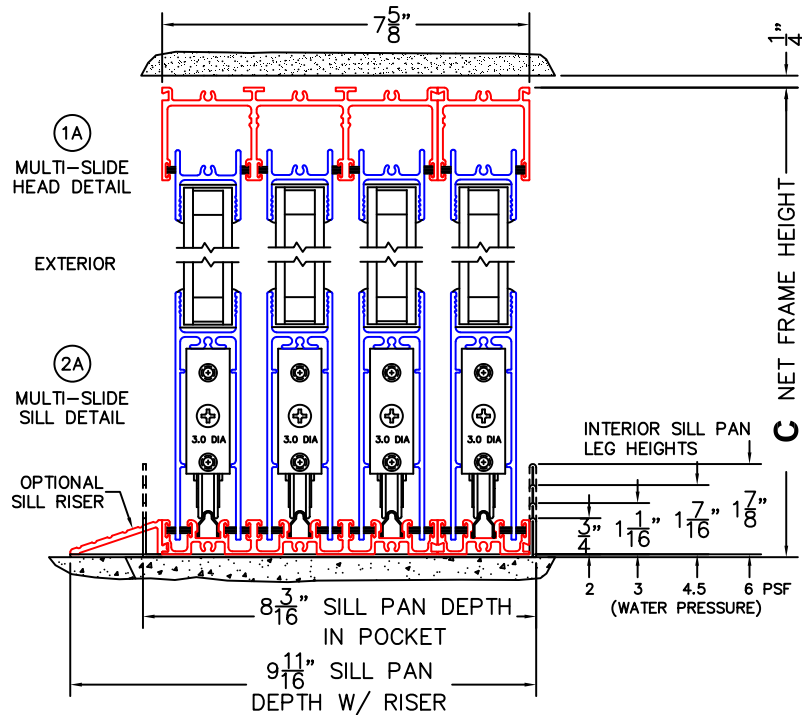
PXIXXXP DOOR SHOWN
