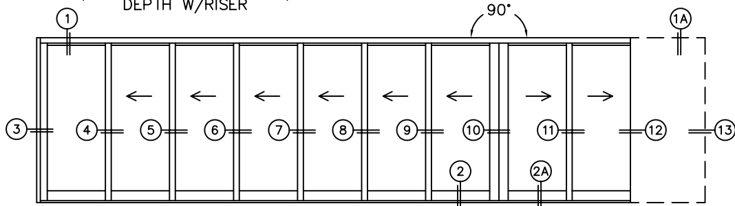
OXXXXXXIXXP DOOR SHOWN
