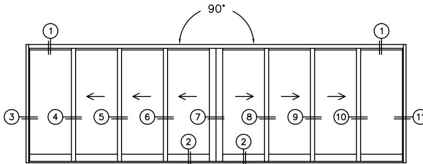
OXXXIXXXO DOOR SHOWN
