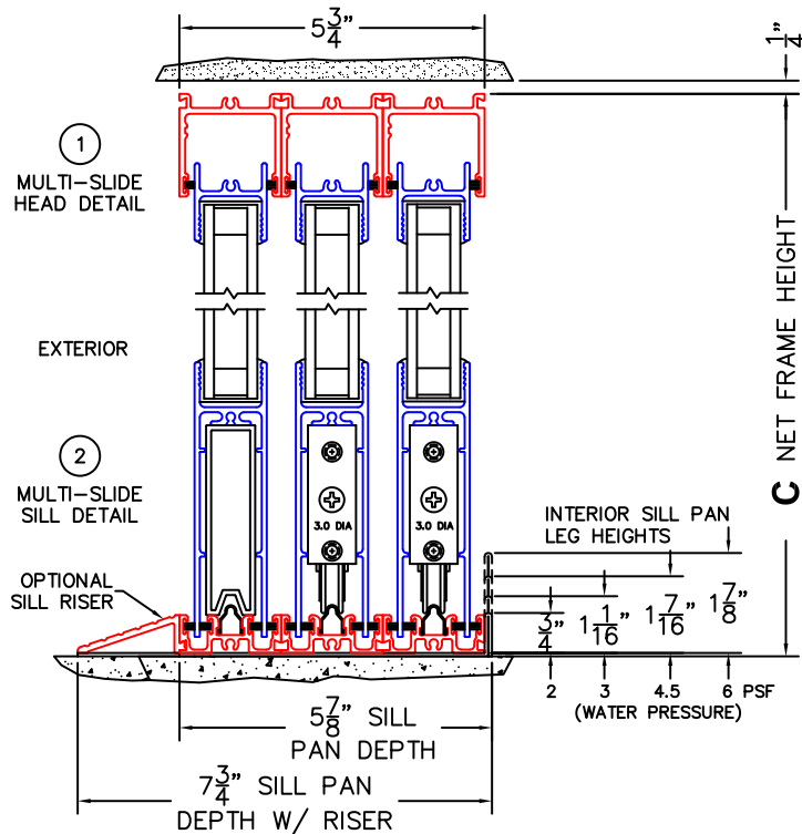
OXXIXX DOOR SHOWN
