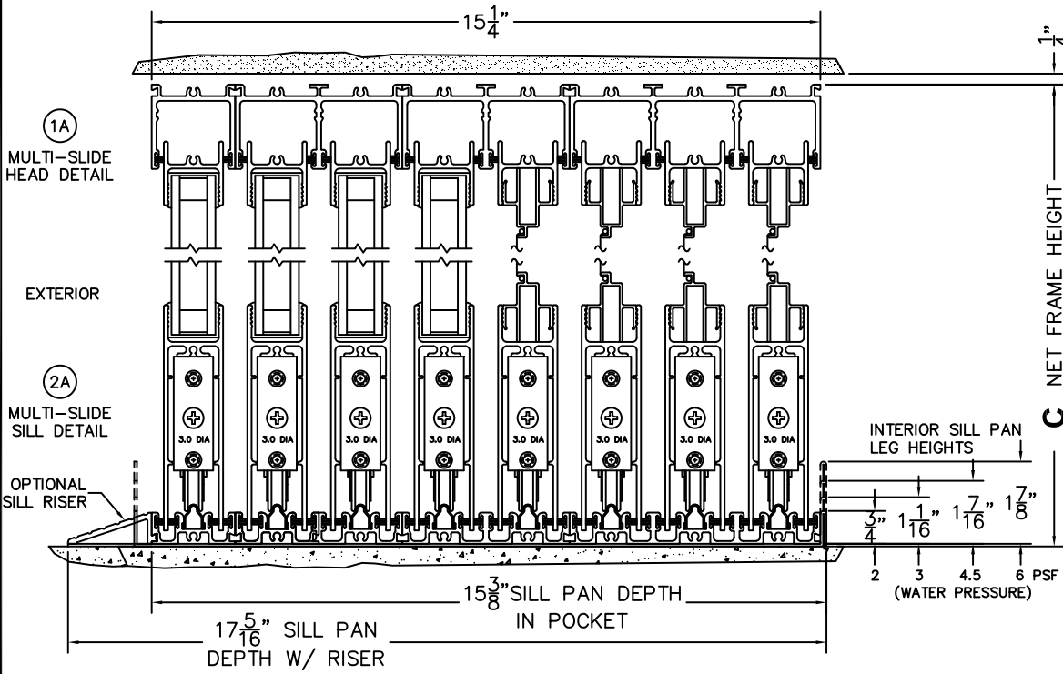
OXIXXXXP DOOR SHOWN
