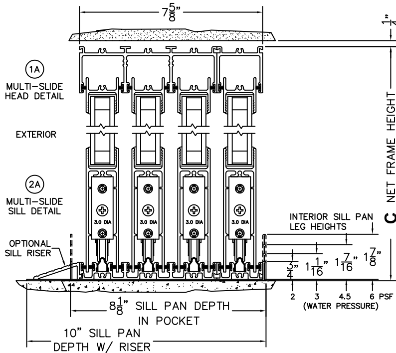
OIXXXP DOOR SHOWN
