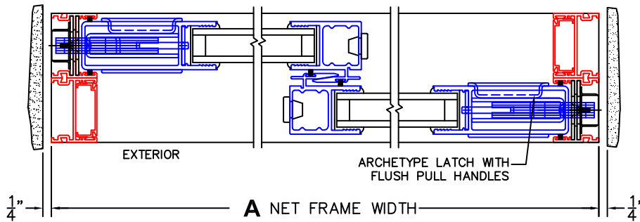
3 LOCK JAMB
