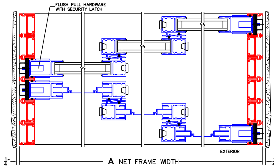
8 LOCK JAMB
