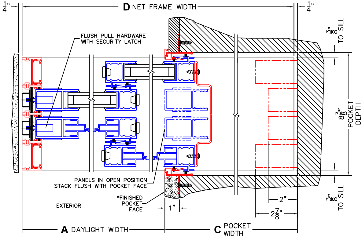
③ LOCK JAMB ④ INTERLOCKERS ⑤ POCKET INTERLOCKER ⑥ POCKET JAMB
