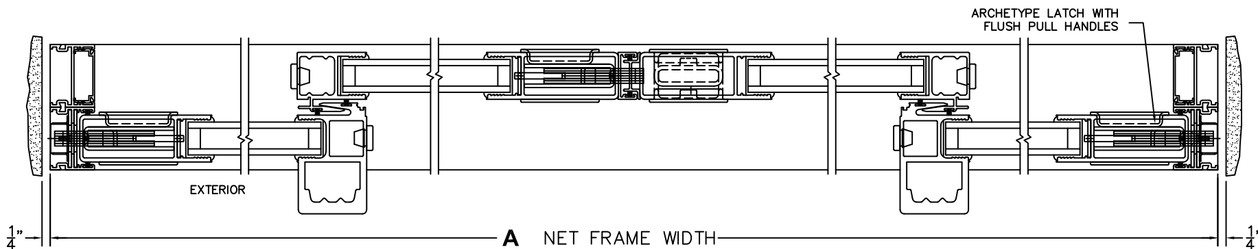
③ LOCK JAMB
