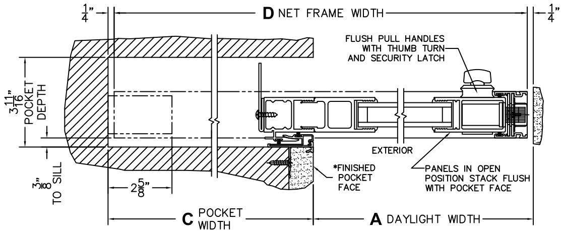
3 POCKET JAMB
