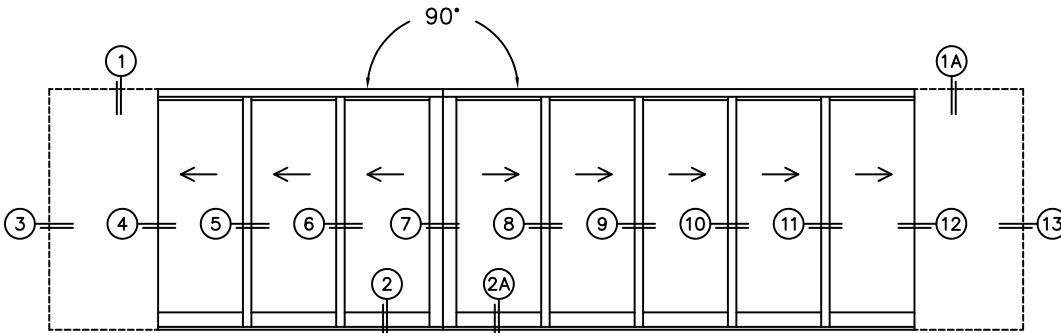
PXXXIXXXXXP DOOR SHOWN
