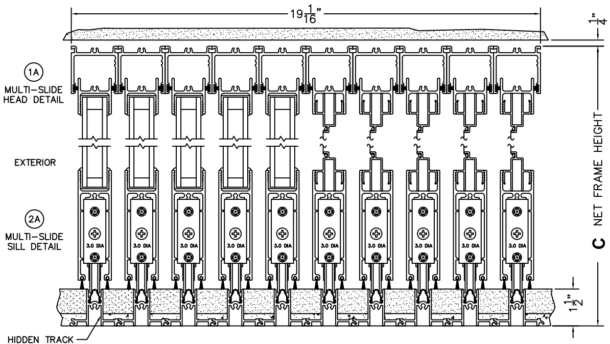
PXXXIXXXXXP DOOR SHOWN
