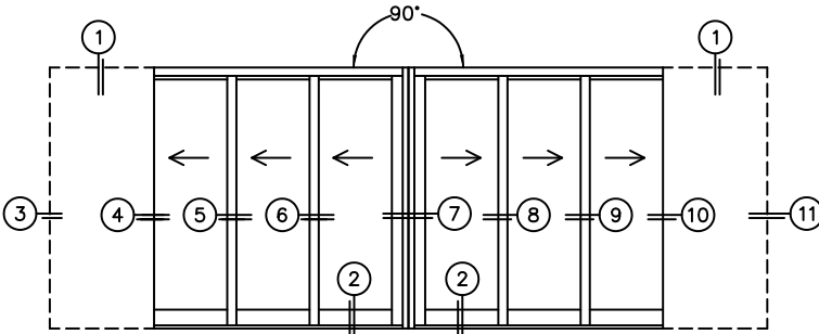
PXXXIXXP DOOR SHOWN
