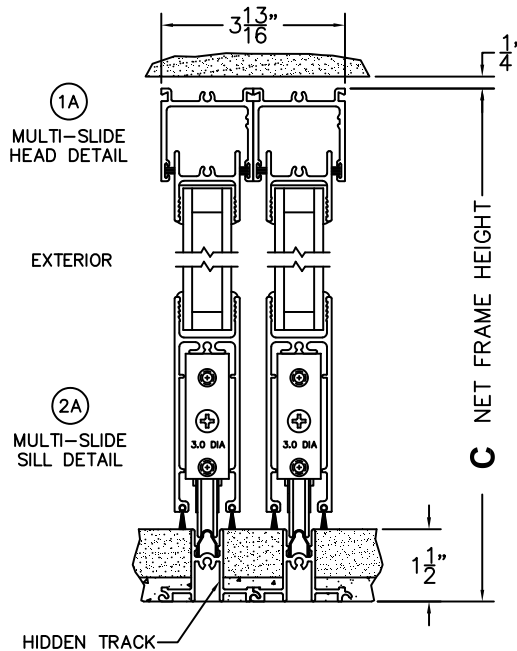
PXXXIXXP DOOR SHOWN
