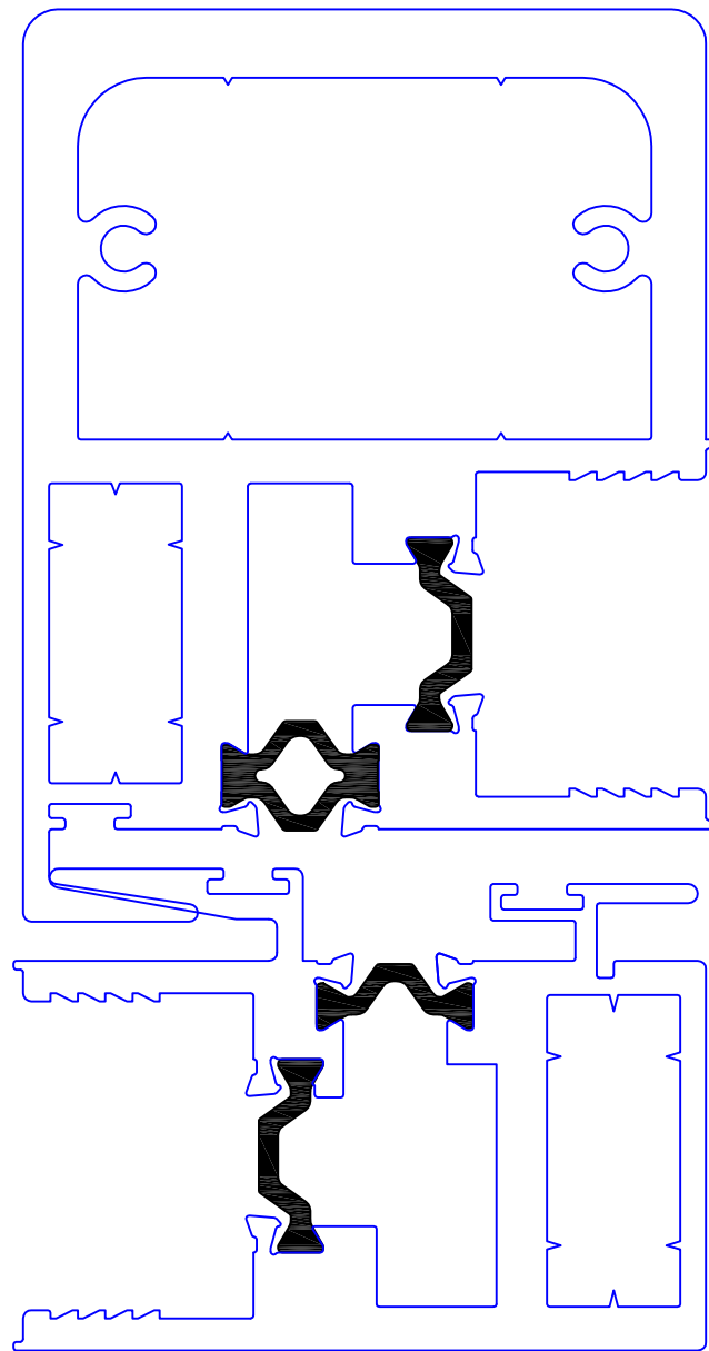
HP. THERMAL INTERLOCKERS
